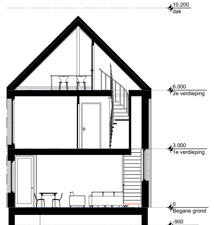
Doorsnede A-A
